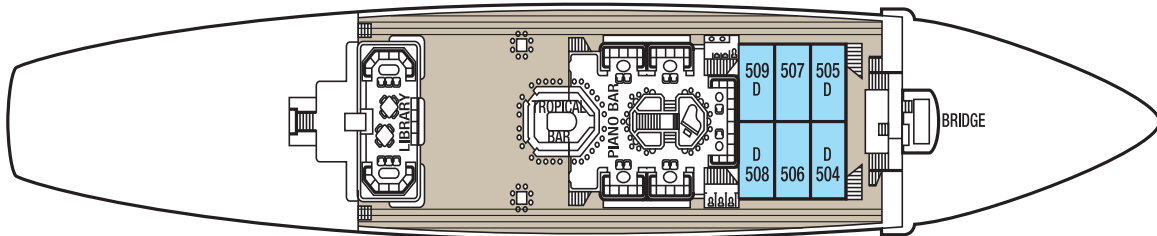
HOOFDDEK
