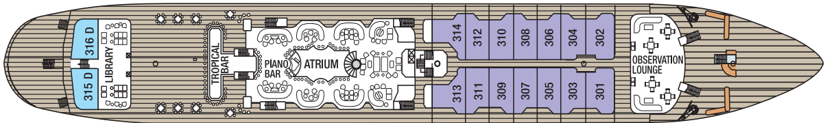
HOOFDDEK
